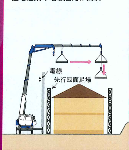
住宅建築の電線越え作業例
