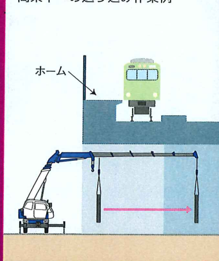
高架下への送り込み作業例
